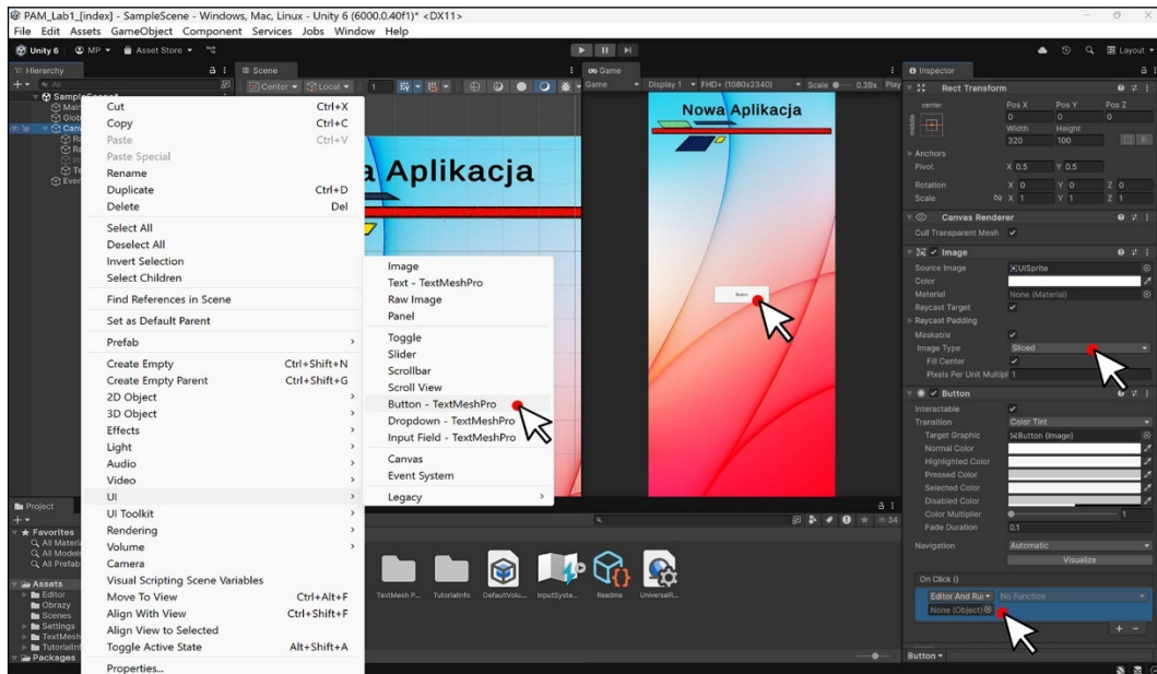
Rys. 27. Ustawienia przycisku
