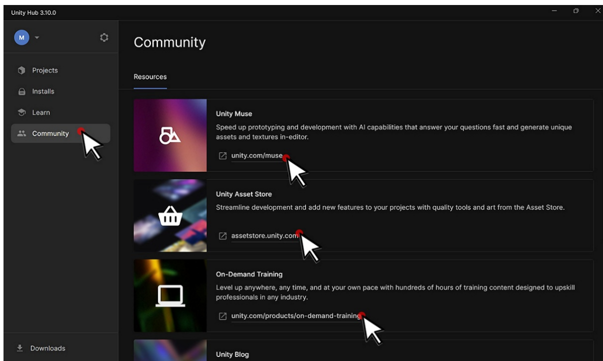
Rys. 9. Zakładka Comunity
