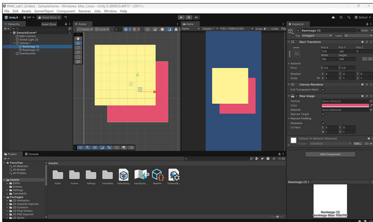
Rys. 21. Warstwy interfejsu
