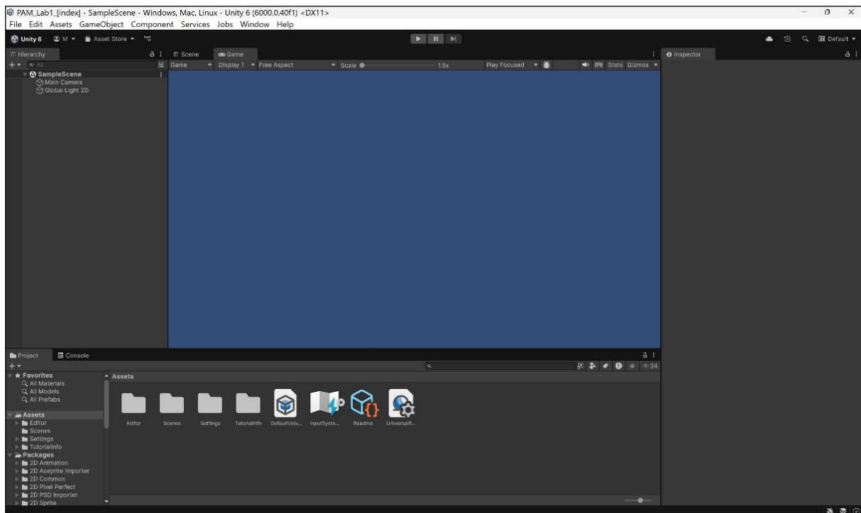
Rys. 13. Okno Game
