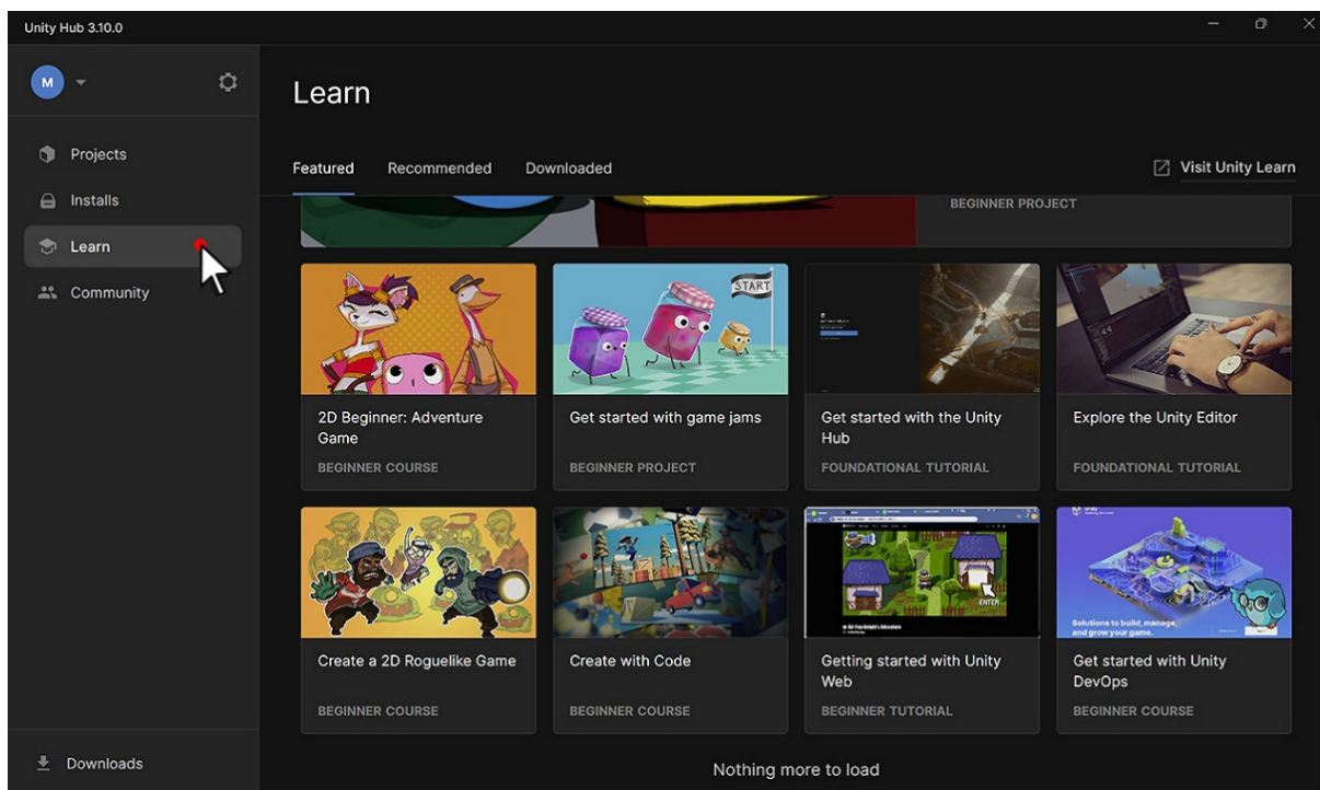
Rys. 8. Zakładka Learn
