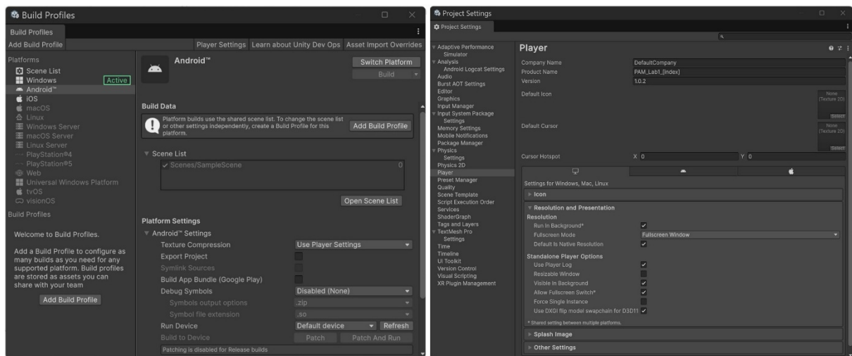
Rys. 31. Ustawienia projektu
